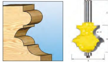
Φρέζα για πολλαπλά προφίλ
