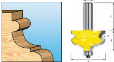
Φρέζα για πολλαπλά προφίλ
