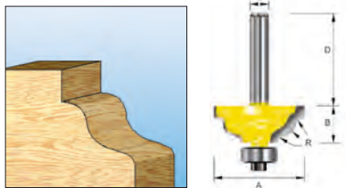
Φρέζα κυματοειδούς προφίλ
