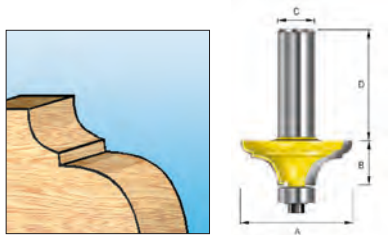
Φρέζα κλασσικού προφίλ
